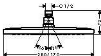
Croma E 280 1jet 26257000 / 26257005 Croma E 280 1jet EcoSmart 26258000 / 26258007
